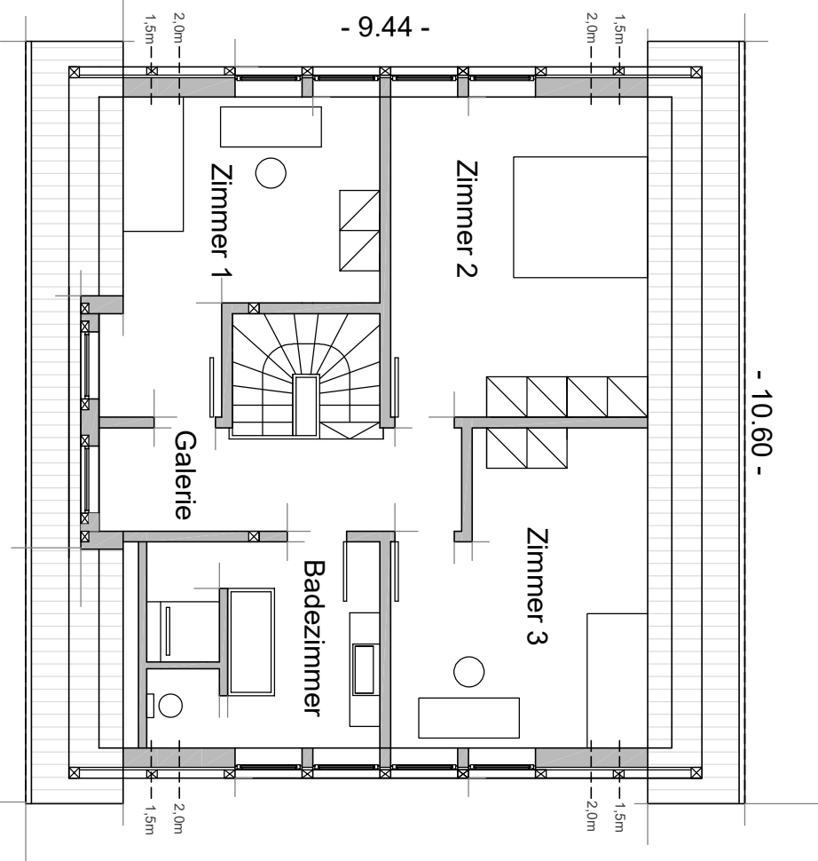
Grundriss Dachgeschoss
