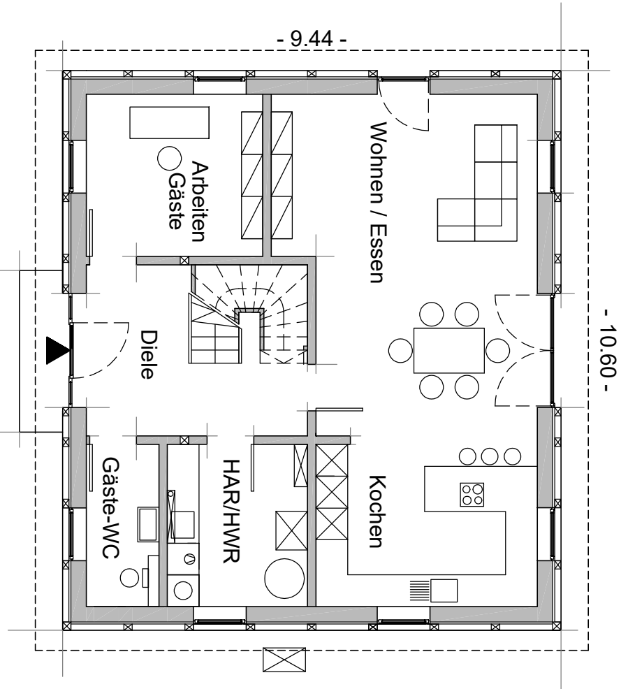
Grundriss Erdgeschoss
